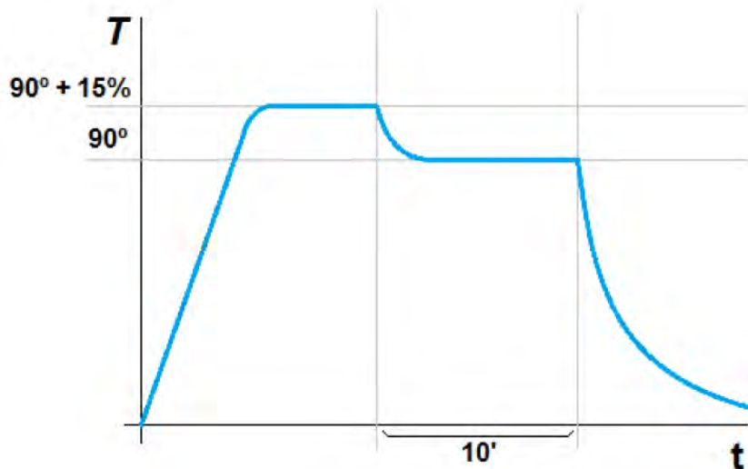
Figura 14. Temperatura horno
