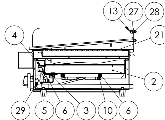
SECCIÓN B-B
